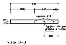
Vista B-B
